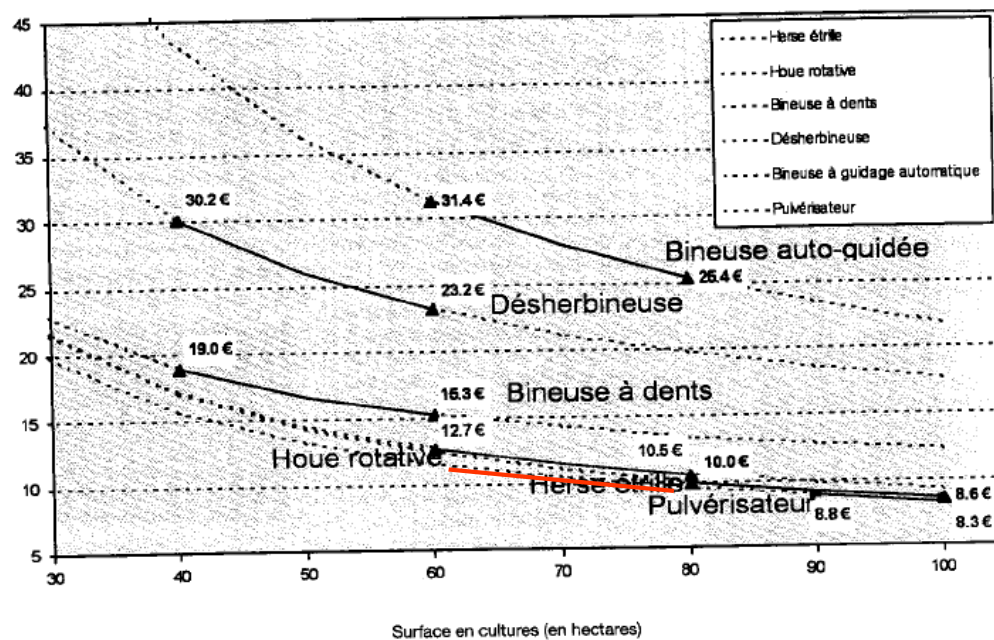
Coûts calculés «matériel + traction» pour 2 passages (sauf pulvérisateur 5 passages)
